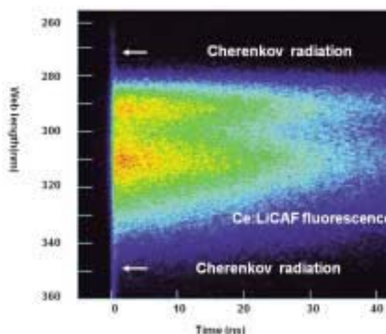
図3 電子ビームで励起したセリウムライカフ結晶からの発光のストリークイメージ。時間を追って波長ごとの強度を測定したもの。290 nm 付近、320 nm 付近のピーク数が数十ナノ秒にわたって持続するのがわかる。
