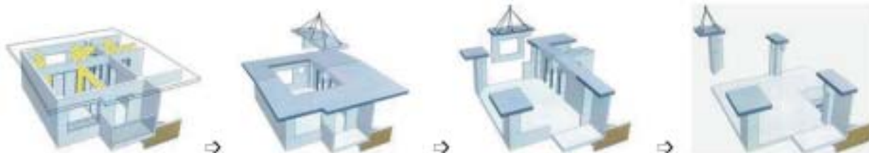
図10 減築の施工手順
