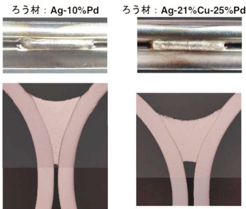
図2 レーザブレイジングによるNi基耐熱合金チューブの管束ろう付 (チューブ肉厚：0.5mm)
