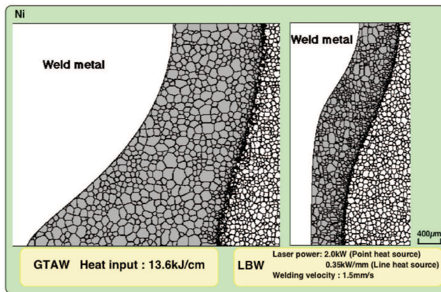
図3 Ni 溶接部の再結晶・粒成長シミュレーション結果（モンテカルロ法）
