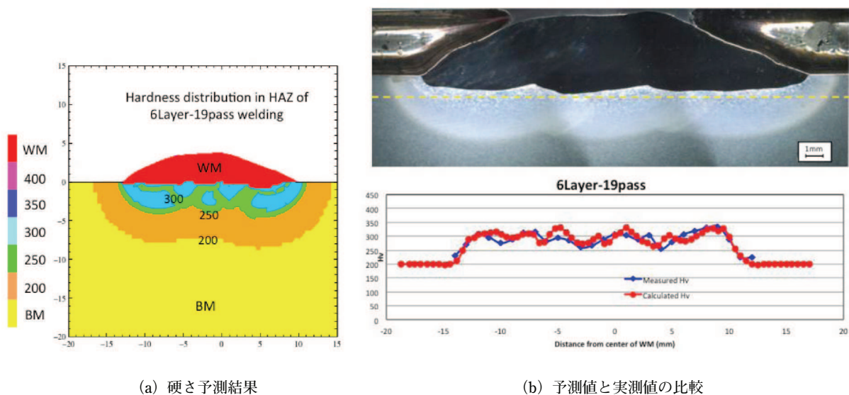
図4 低合金鋼テンパービード溶接部の硬さ予測結果
