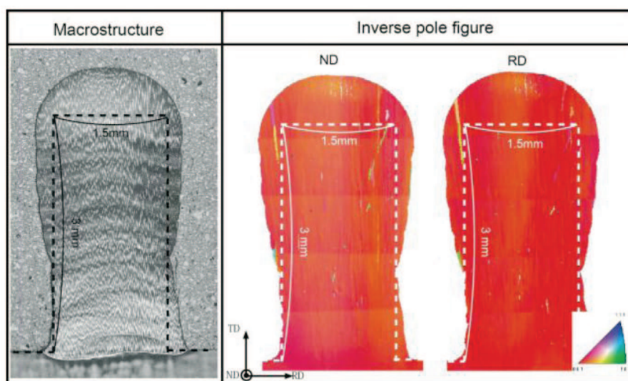
図1 Ni基単結晶合金に対するレーザー単結晶肉盛の断面組織と結晶方位解析結果
